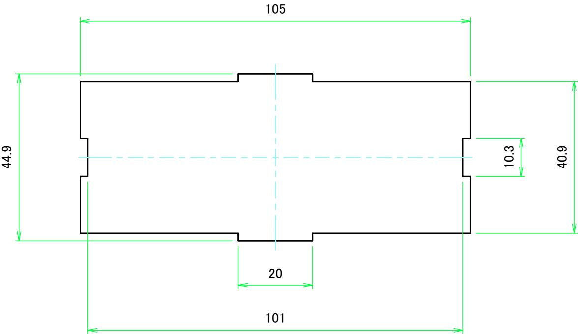
Wパネル1表面 / W Panel 1 Frontside
