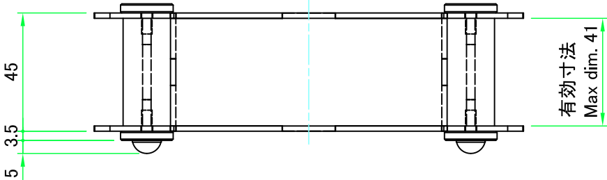
Wパネル1 / W Panel 1
